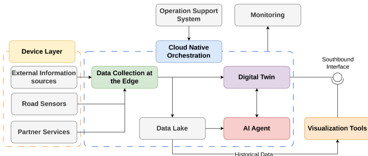
Figura 7 - Componentes arquitetônicos.
